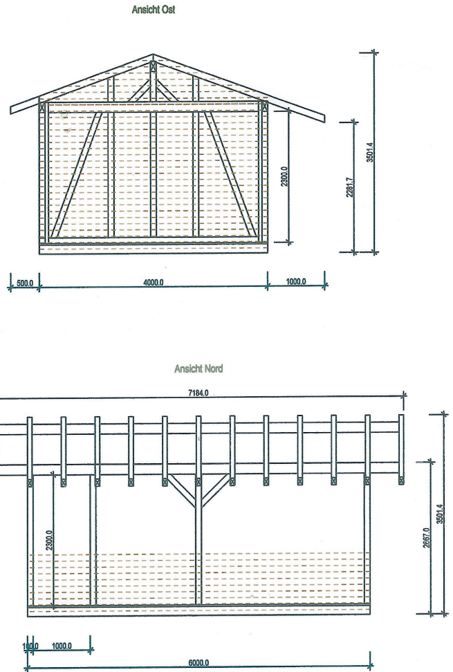
Planskizzen des Infopoints
